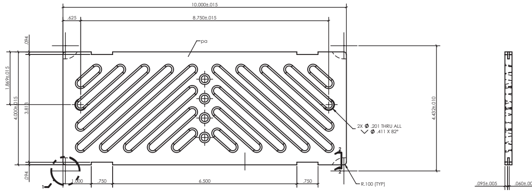
DETAIL: SVI-4x10
