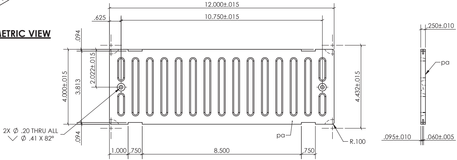
DETAIL: SVI-4x12-F
